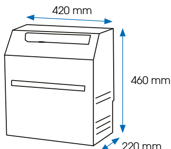
Kompressordel luftkjølt
